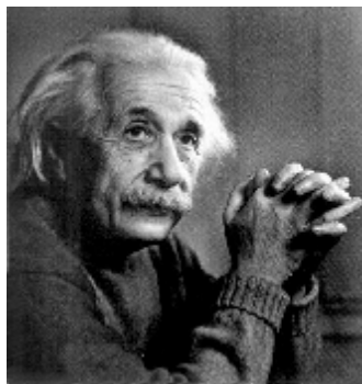
Albert Einstein
